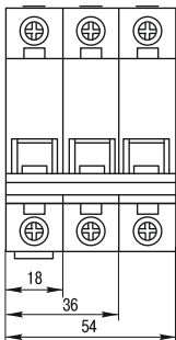
Рисунок 4 – Основные размеры
