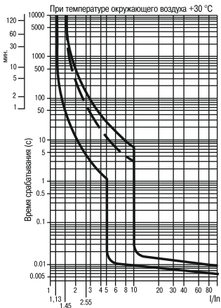
Рисунок 1 – Пунктирная линия – верхняя граница время-токовой характеристики для автоматических выключателей с номинальным током I_n \leq 32 А.
