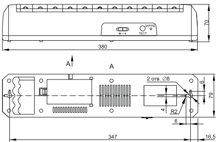
Рисунок 5 – ДБА 3928, ДБА 3928-П
