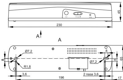
Рисунок 3 – ДБА 3926, ДБА 3926-П
