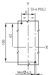
3 Разделительная пластина
