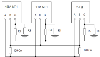
Рисунок 2.1 – Схема подключения счетчиков к интерфейсной линии EIA-485
