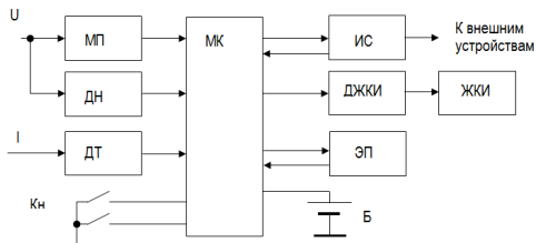
Рисунок 1.2 – Функциональная схема счетчика
