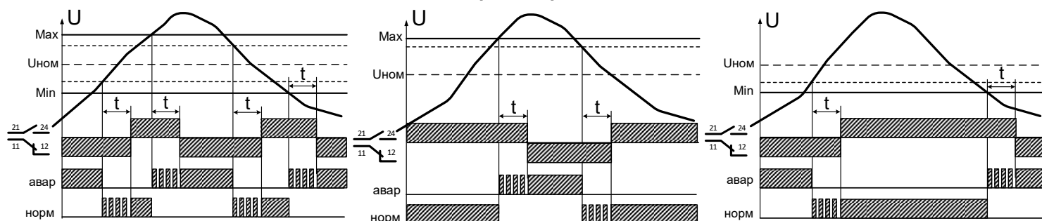
Рис. 2а. Реле напряжения "работа «окном»"
