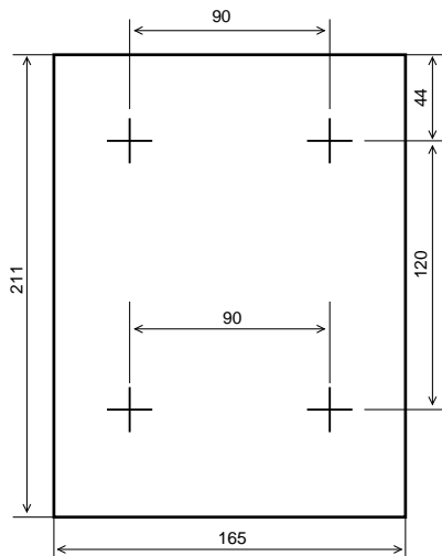
Рисунок 2. Габаритно-установочные размеры
