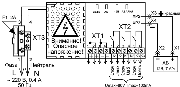
Рисунок 3. Схема подключения РИП-12 исп.14 (РИП-12-2/7П2-Р)
