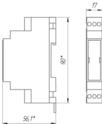
Рисунок 1. Габаритные размеры
