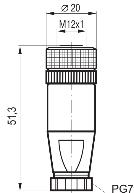
Габаритный чертеж
