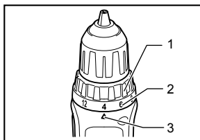
1. Регулировочное кольцо 2. Градуировка 3. Указатель
