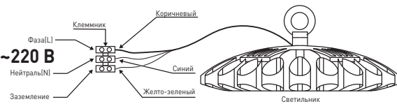
Рис. 1. 220В шамчыракты токто туташтыруу схемасы
