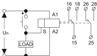
Рисунок 3 – Возможность подключения нагрузки к контактам S-A2
