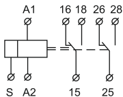
Рисунок 2 – Схема электрическая реле
