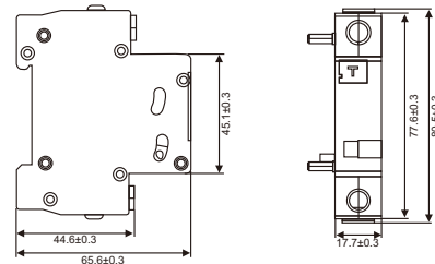
Рисунок 1. Габаритные и установочные размеры
