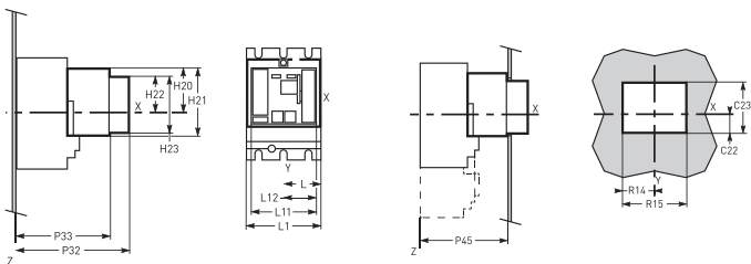
Габаритные и установочные размеры
